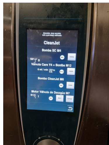
COMPROBACIÓN DE FUNCIÓN CLEANJET
